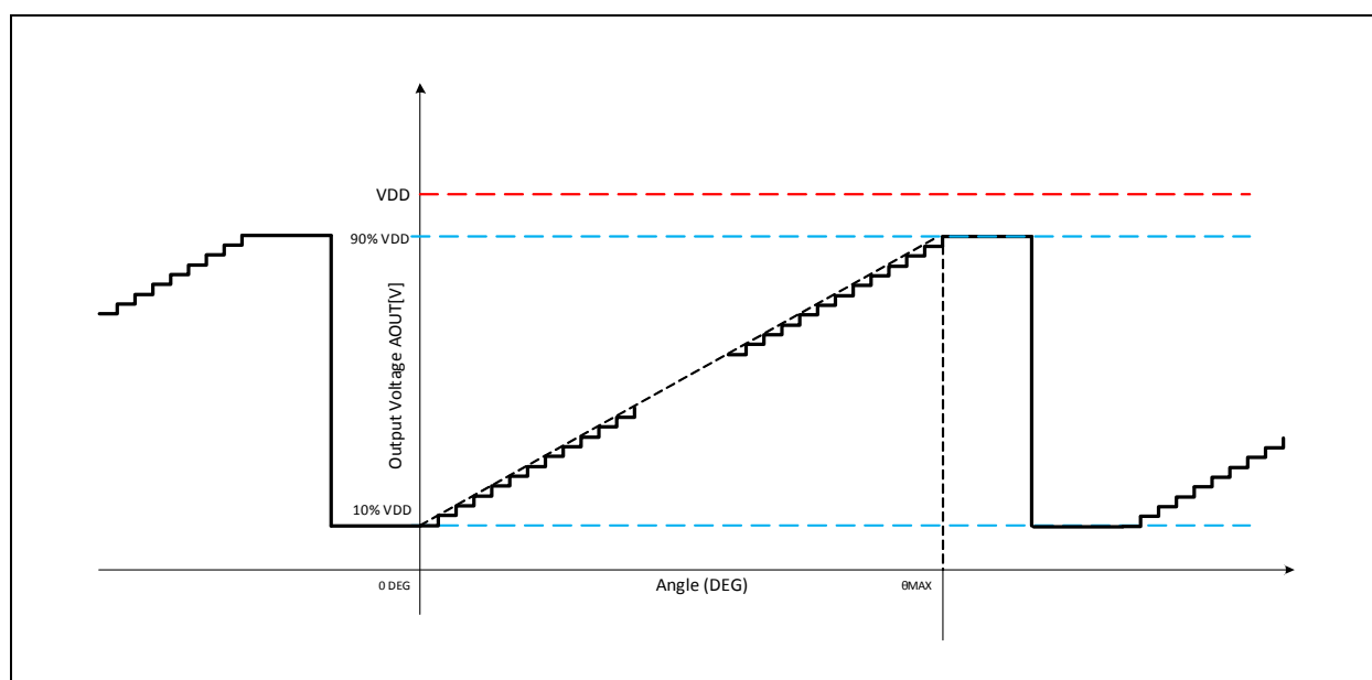
图表 29: 减小输出值的输出特性(10%-90%)
