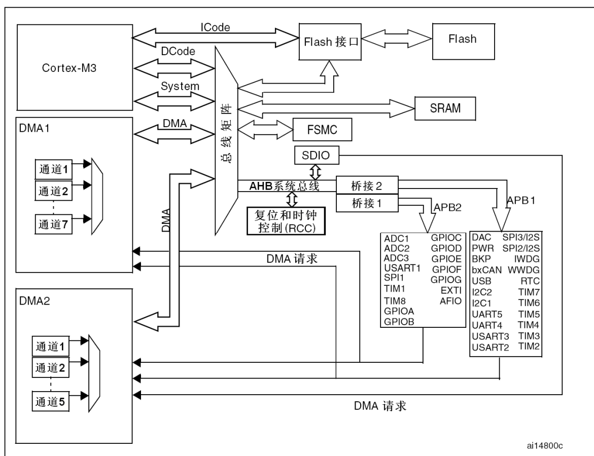
图1 系统结构
