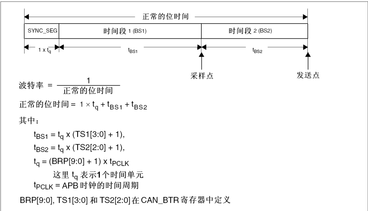
图206 位时序
