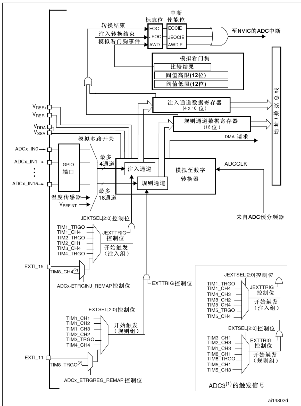
图24 单个ADC框图
