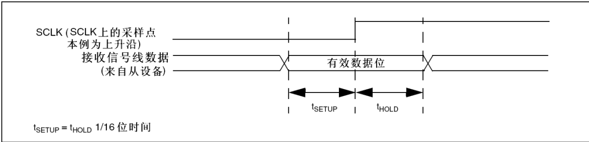
图261 RX数据采样/保持时间
