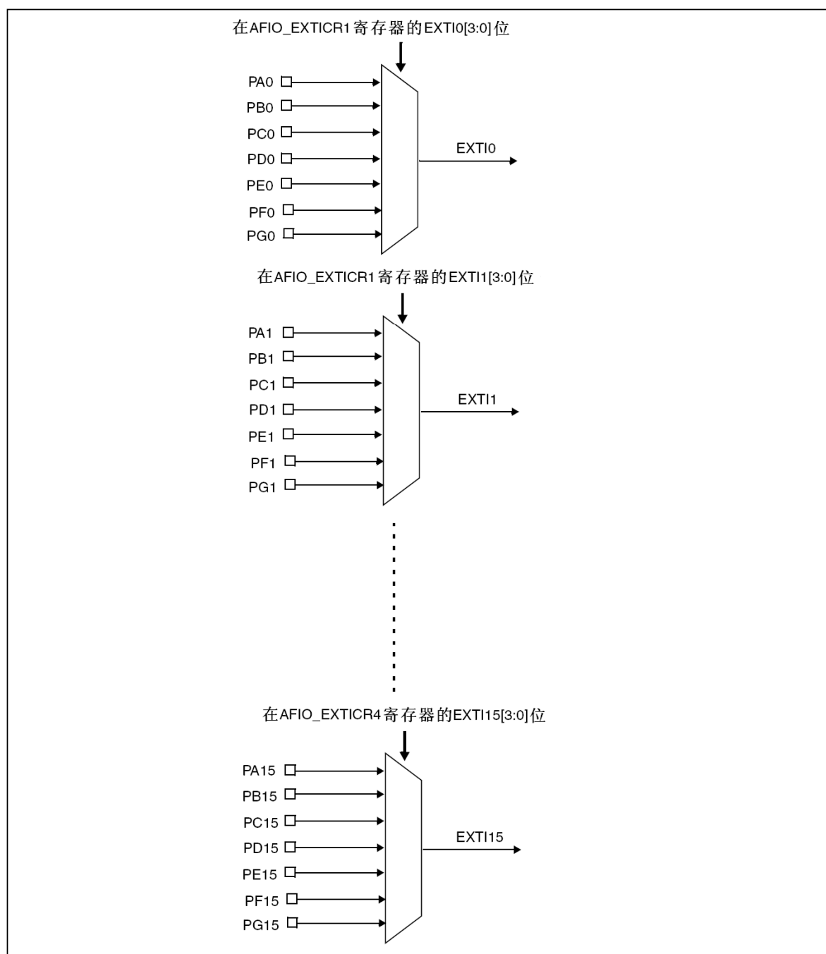
图20 外部中断通用I/O映像
