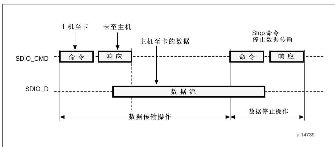
图183 SDIO连续写操作
