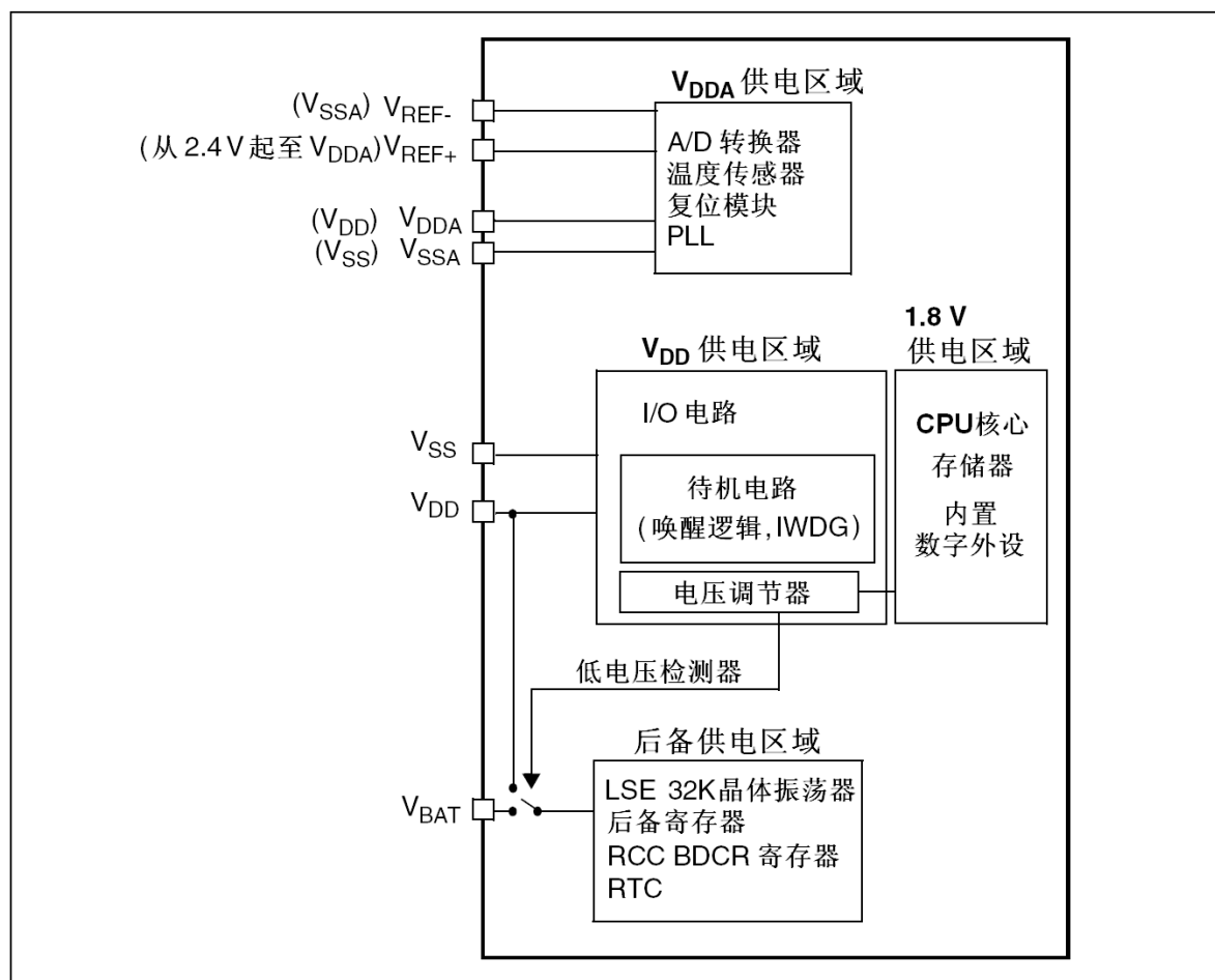
图4 电源框图
