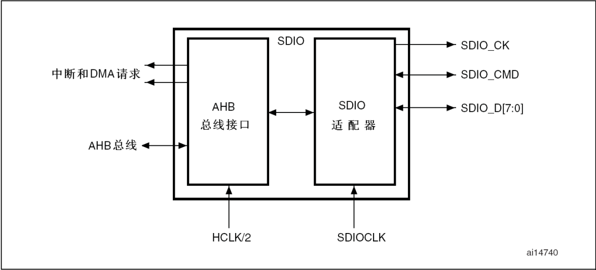
图184 SDIO框图
