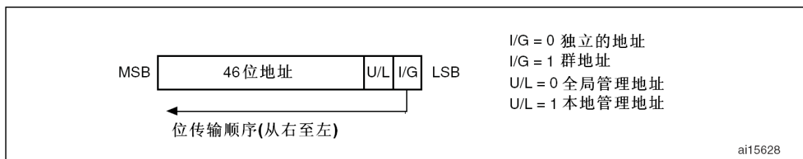
图305 地址域格式
