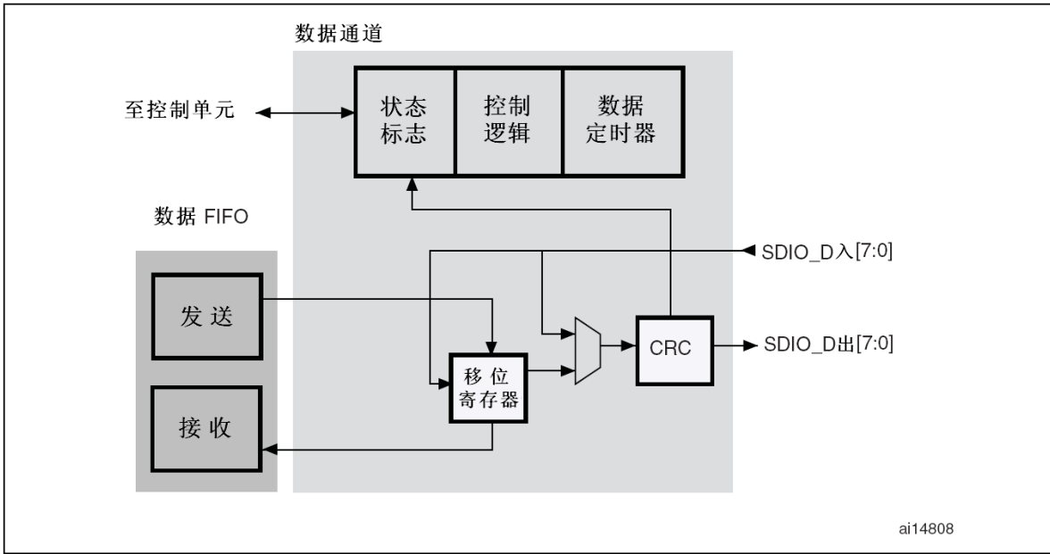
图190 数据通道
