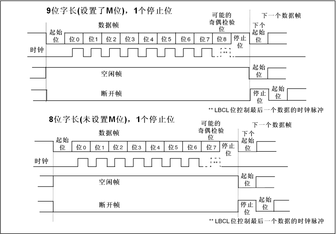
图249 字长设置
