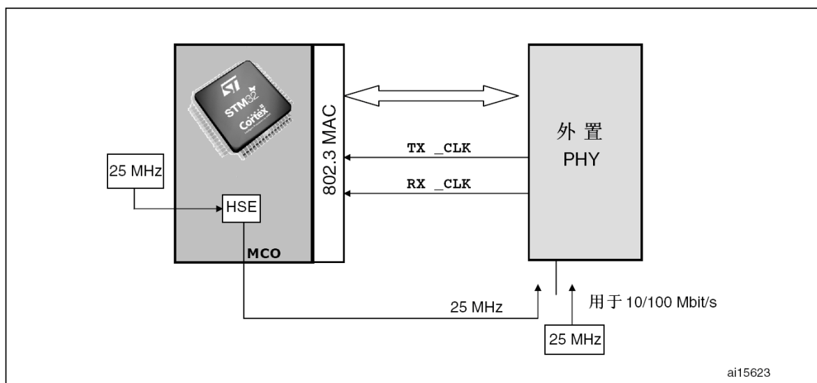
图301 MII时钟源
