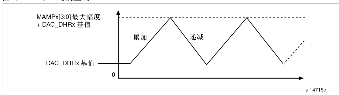
图49 带三角生成的 DAC 转换(使能软件触发)
