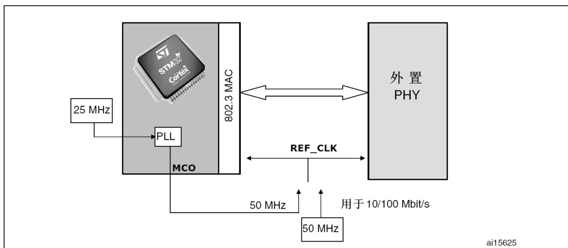
图303 RMII时钟源
