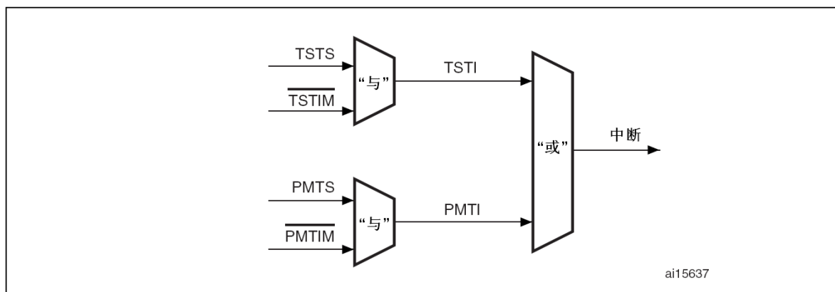
图316 MAC控制器中断屏蔽示意图
