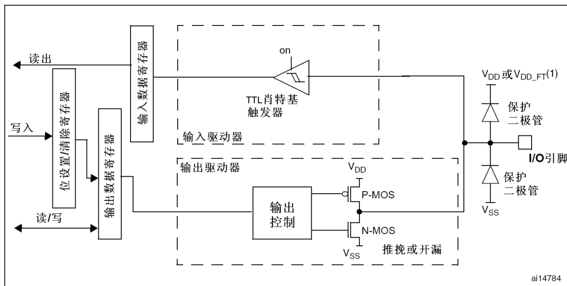
图16 输出配置
