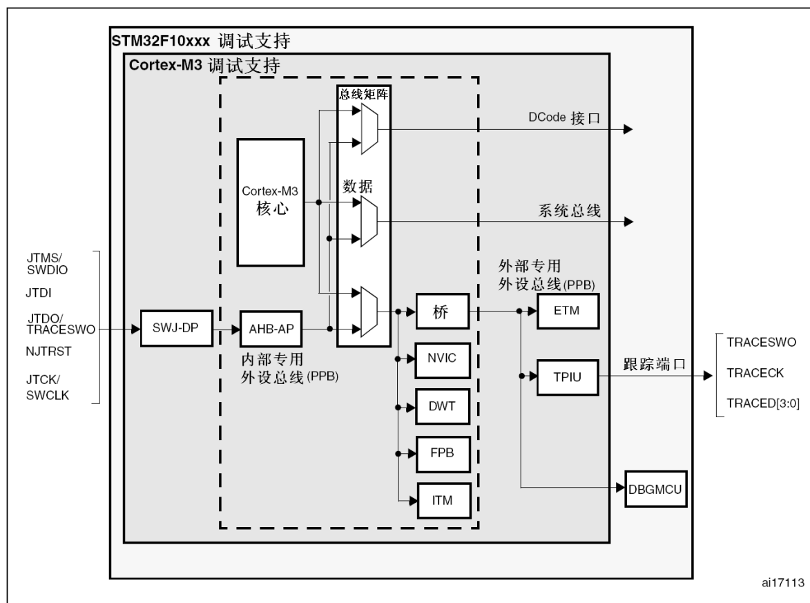
图332 STM32F10xxx级别和Cortex™-M3级别的调试框图
