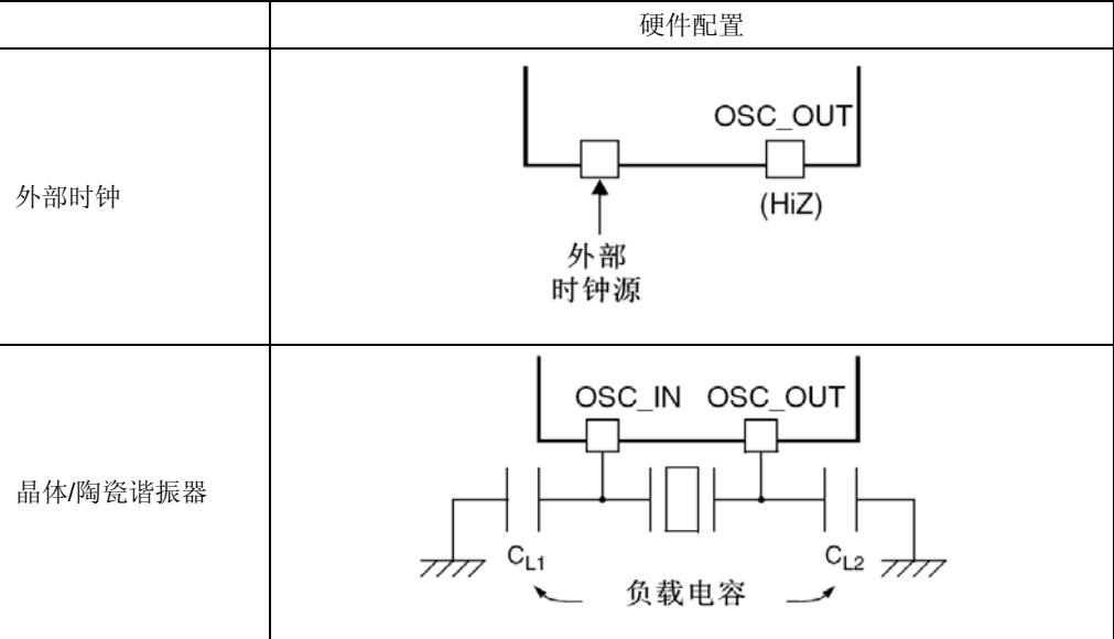
图9 HSE/LSE时钟源
