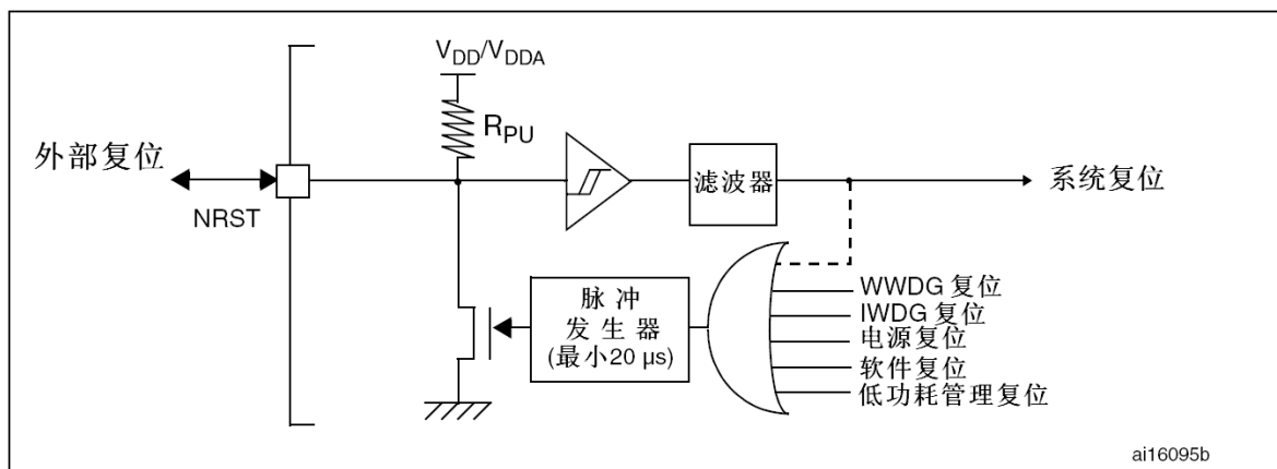
图10 复位电路
