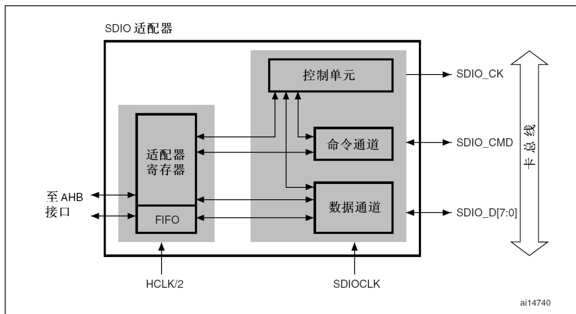
图185 SDIO适配器
