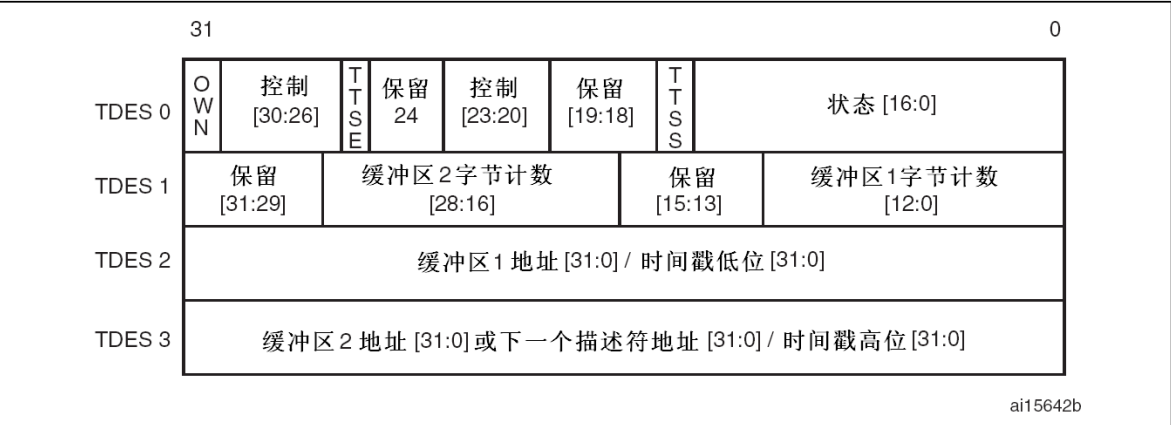
图325 传输描述符
