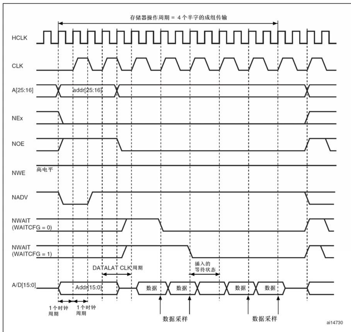
图175 同步的总线复用读模式 – NOR, PSRAM(CRAM)
