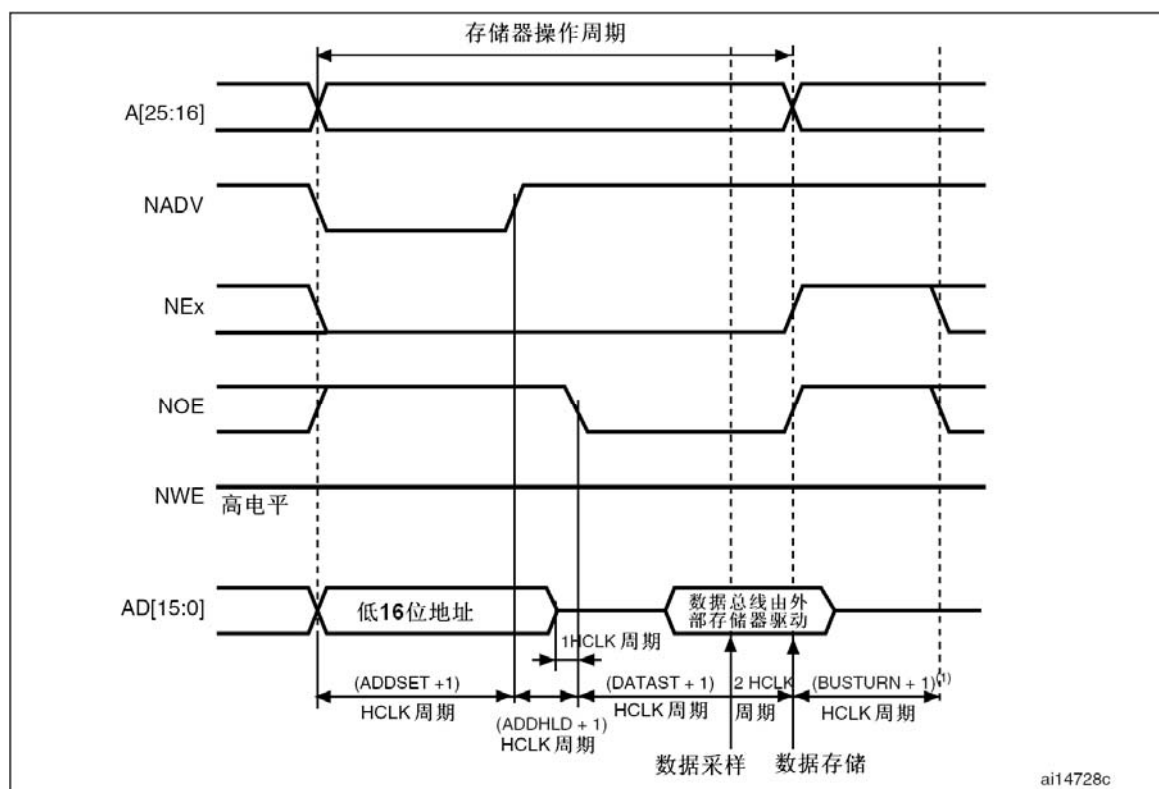
图173 复用读操作
