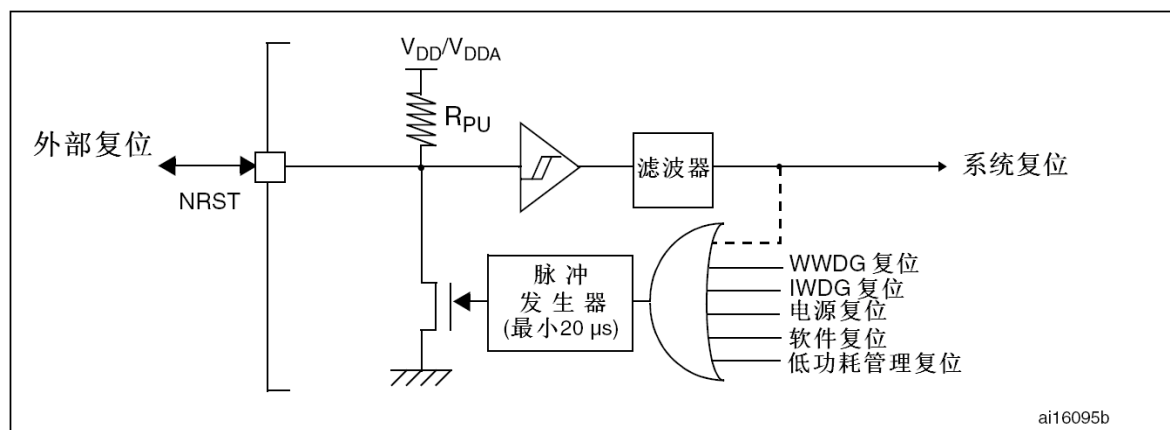
图7 复位电路
