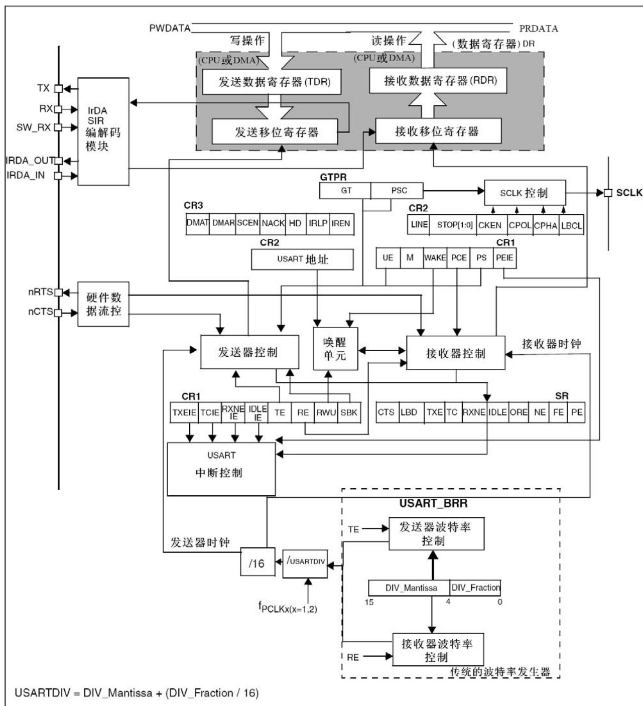
图248 USART框图
