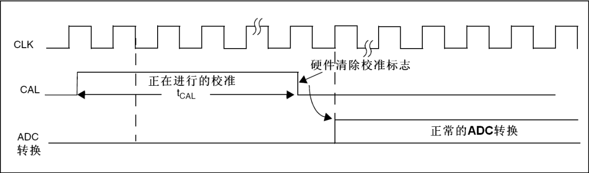
图28 校准时序图
