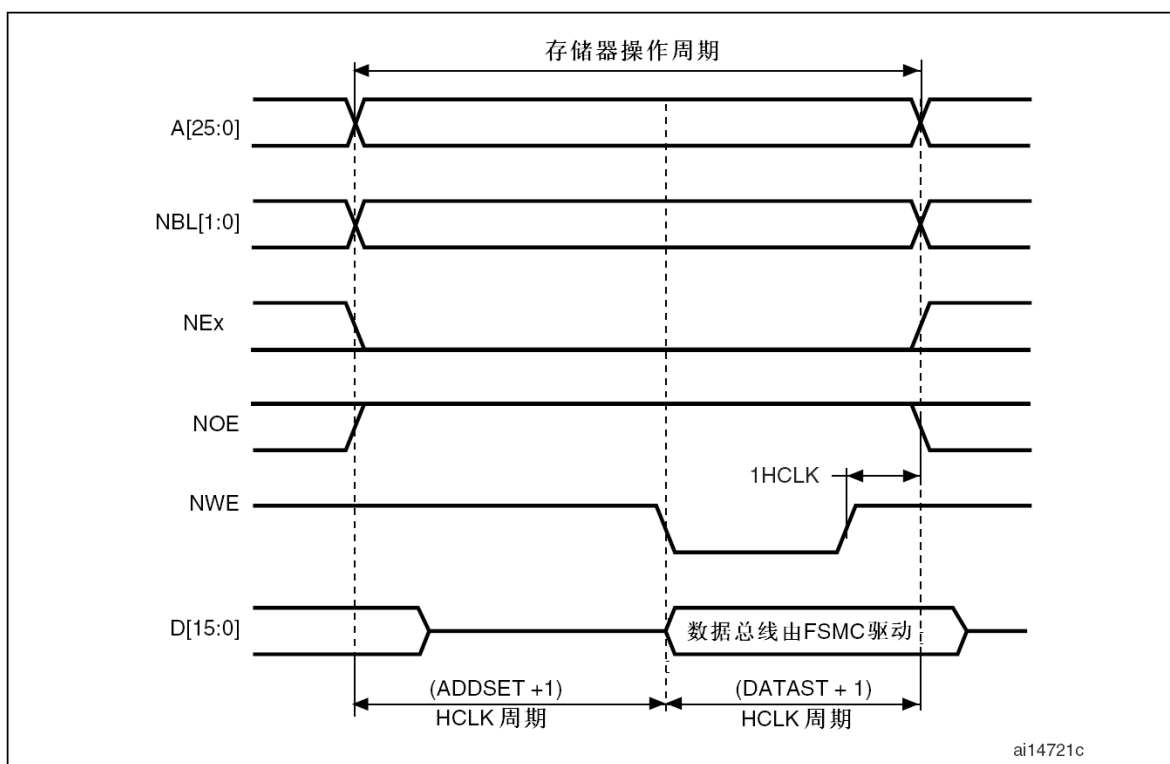
图163 模式1写操作
