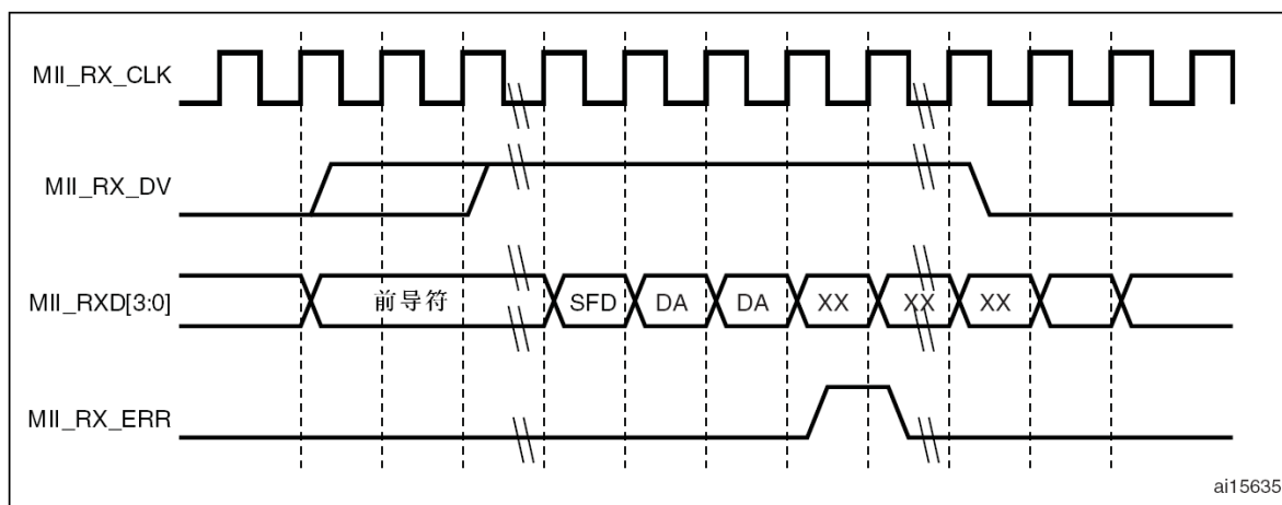
图314 接收时有错误
