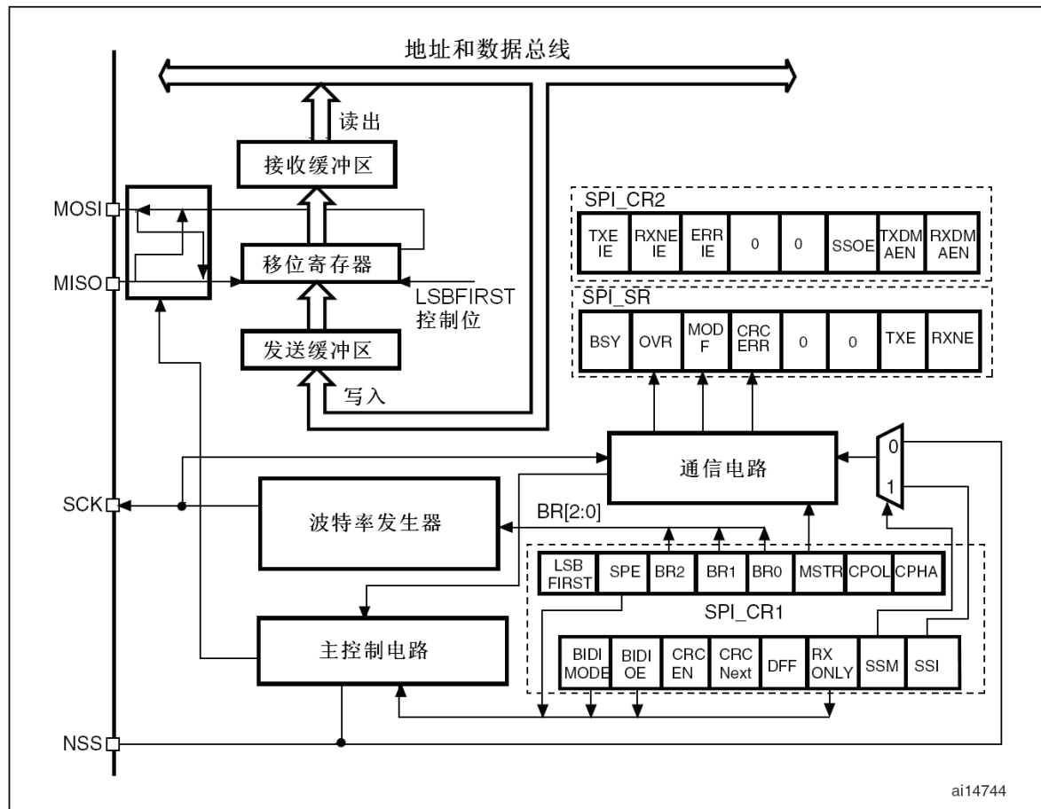
图209 SPI框图
