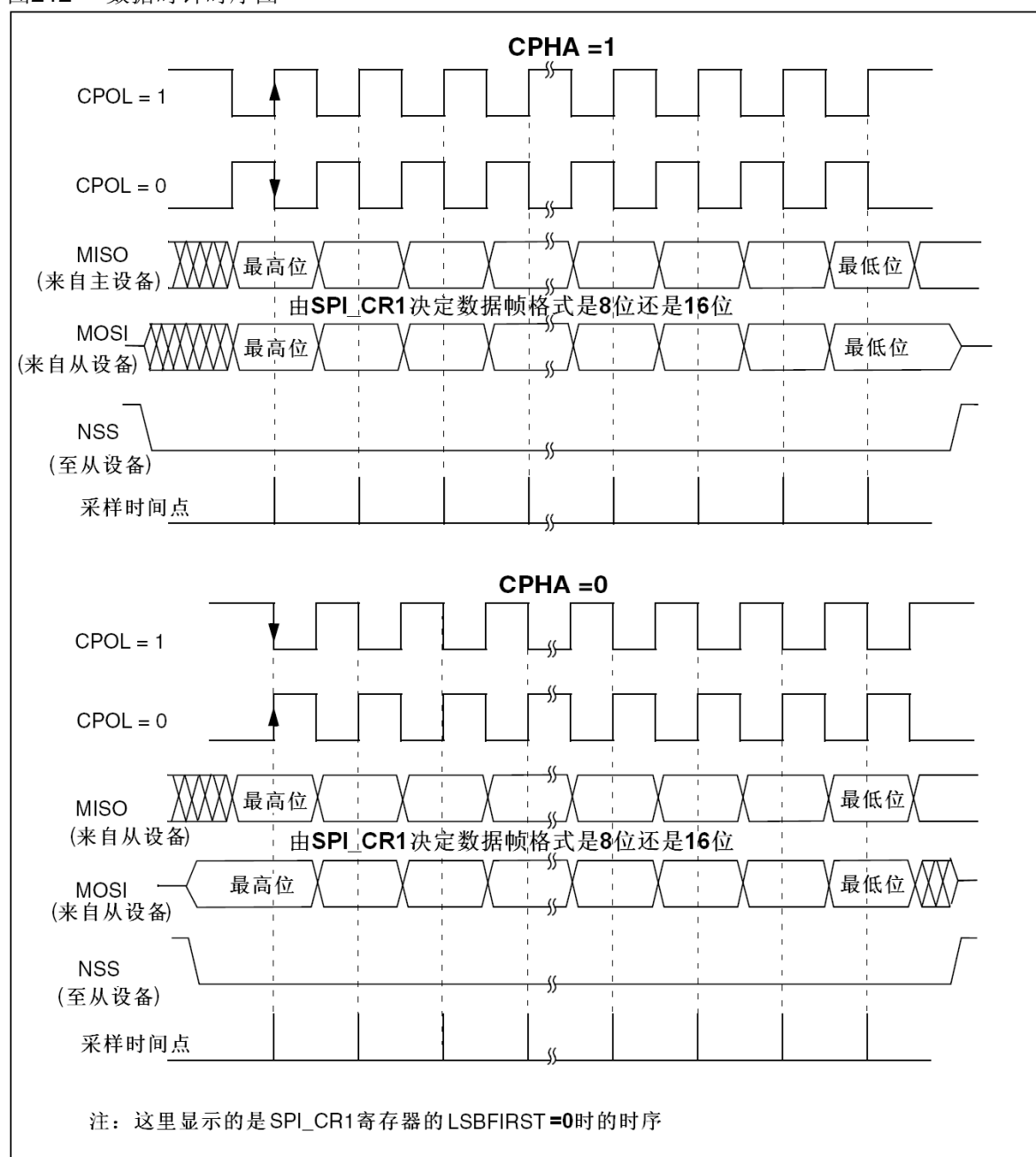
图212 数据时钟时序图
