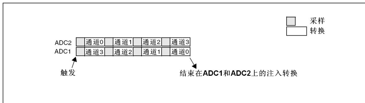
图32 在4个通道上的同步注入模式
