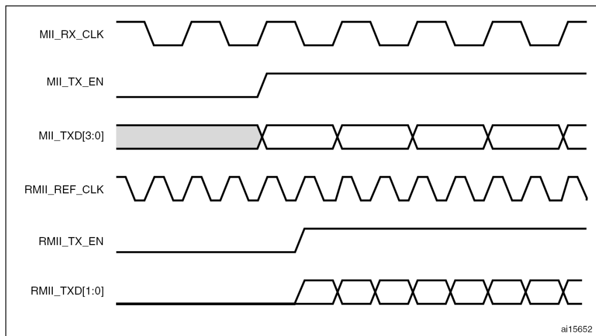
图311 MII和RMII模式下的帧传输
