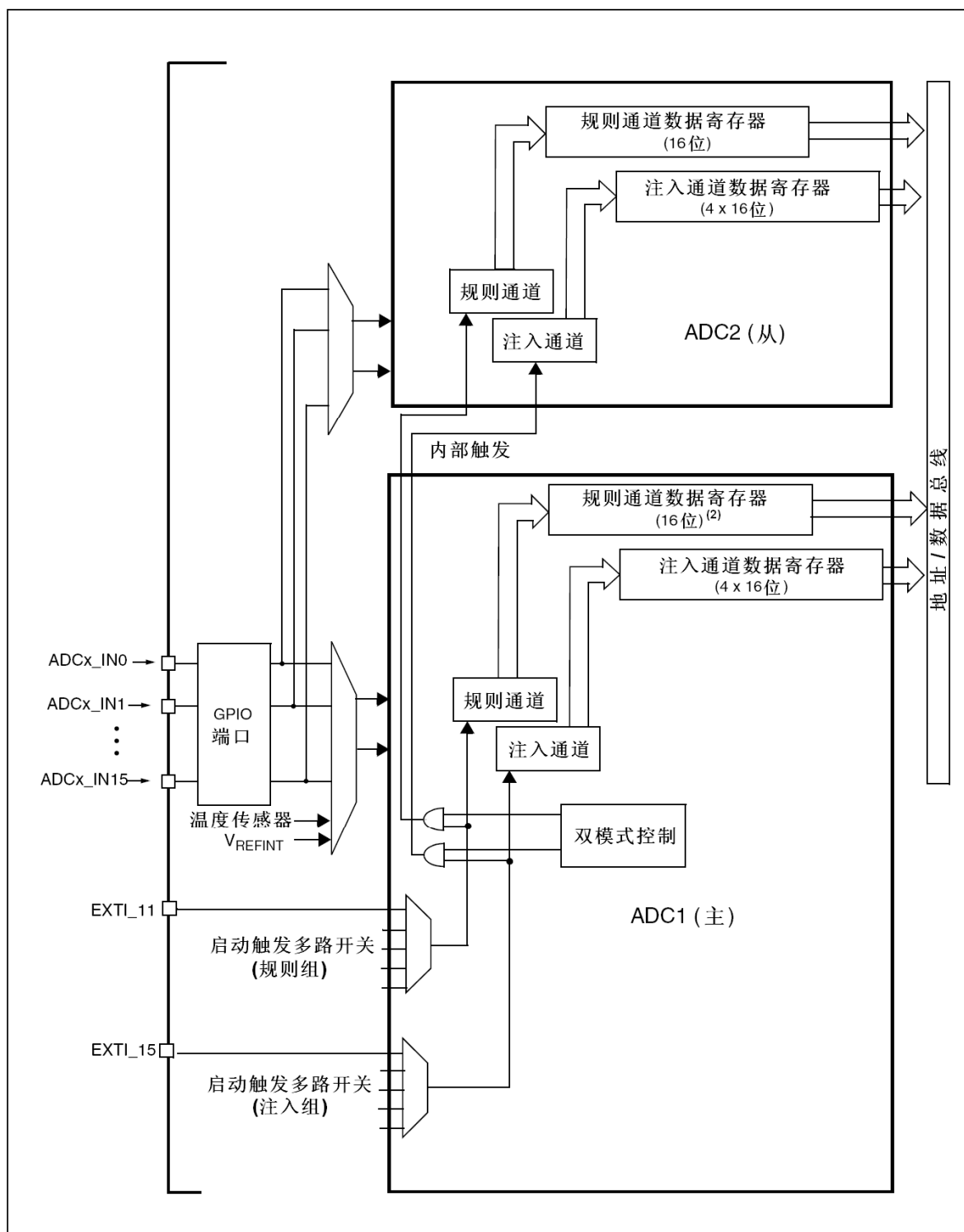
图31 双ADC框图 (1)
