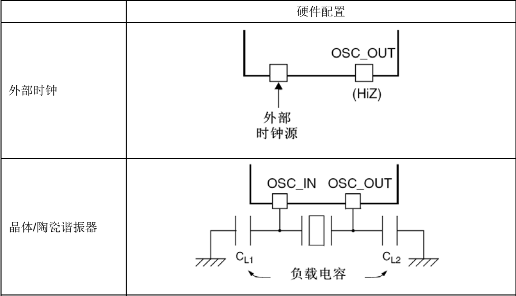
图12 HSE/LSE时钟源
