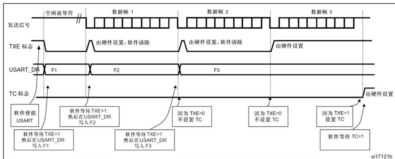
图251 发送时TC/TXE的变化情况
