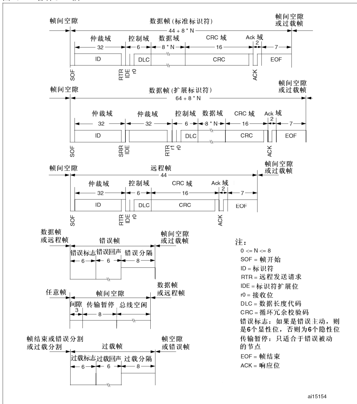
图207 各种CAN帧
