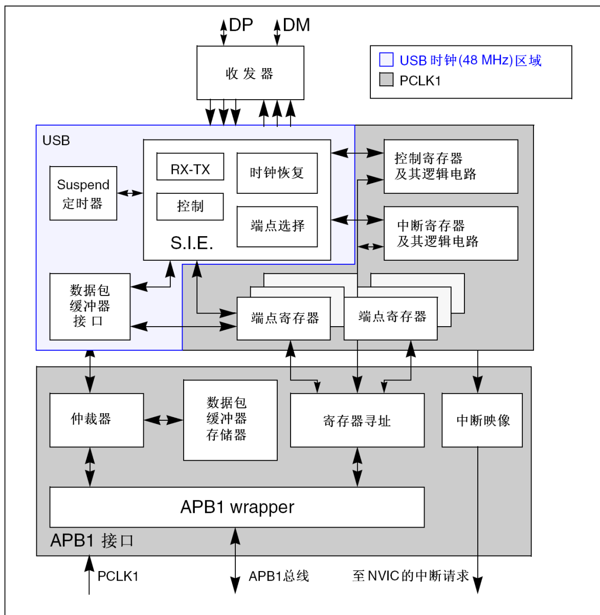
图192 USB设备框图
