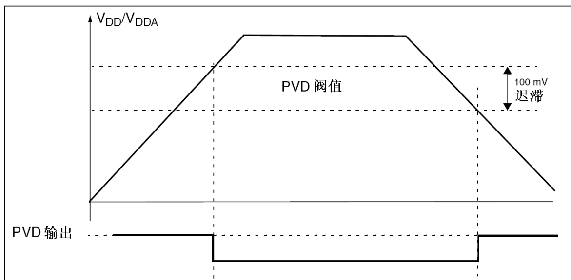
图6 PVD的门限
