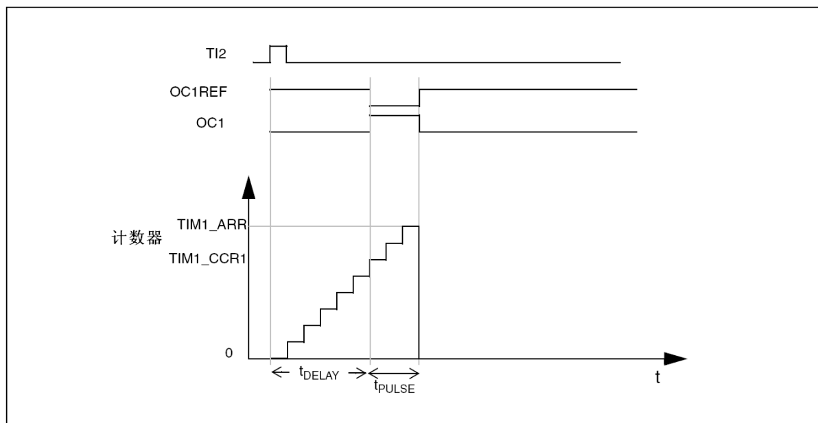
图130 单脉冲模式的例子
