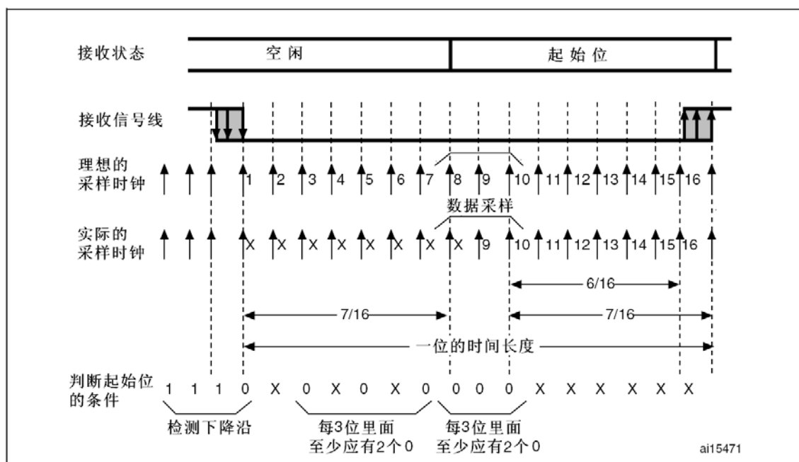
图252 起始位检测
