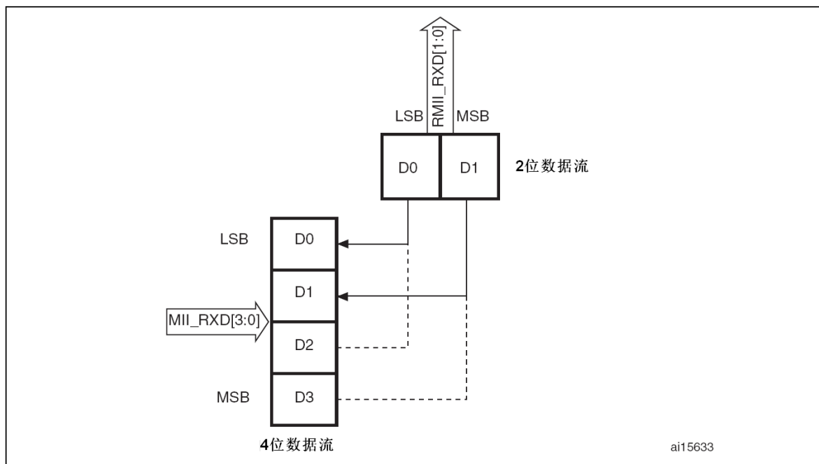
图313 接收时无错误
