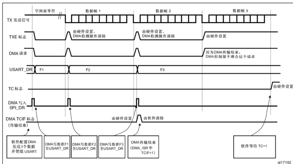
图266 利用DMA发送
