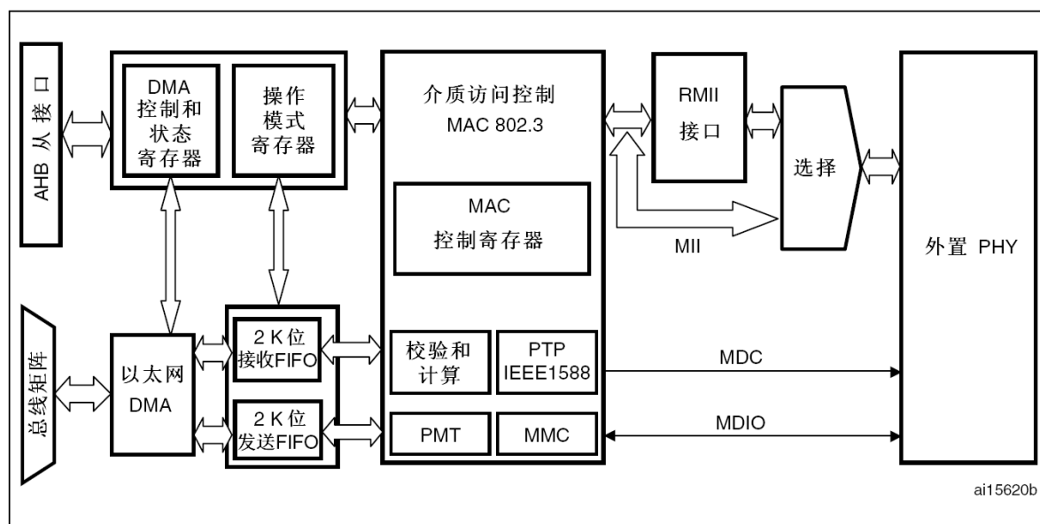
图296 ETH框图
