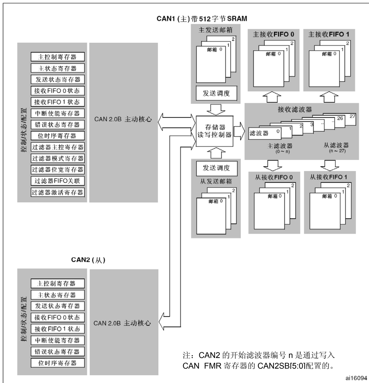
图195 双CAN框图(互联型产品)
