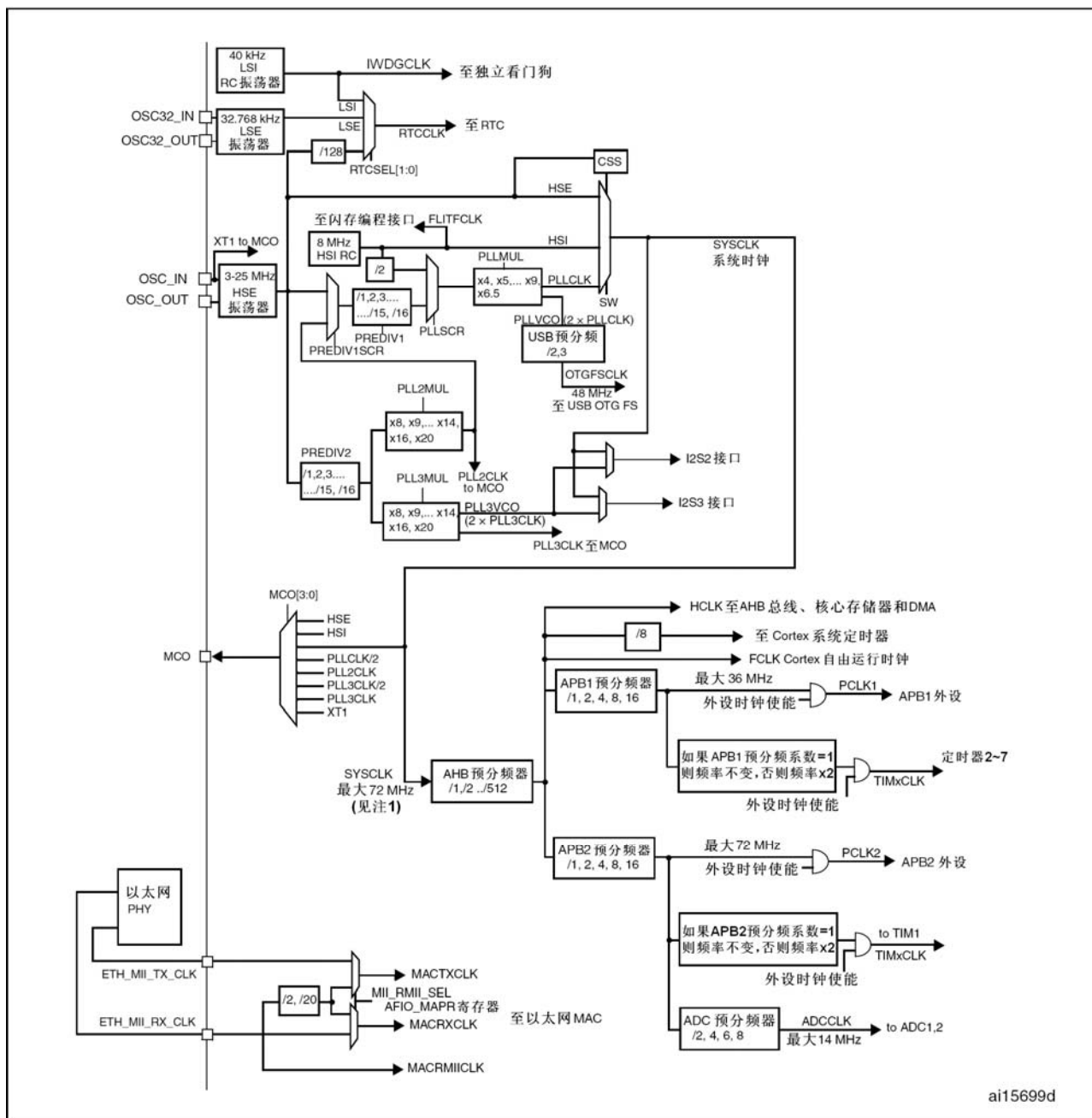
图11 时钟树
