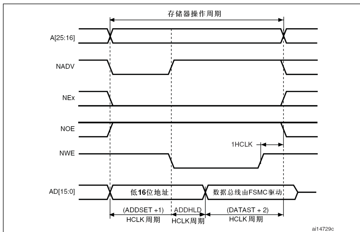
图174 复用写操作
