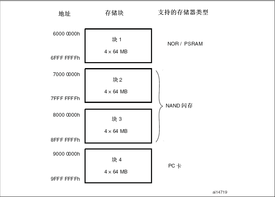
图161 FSMC存储块
