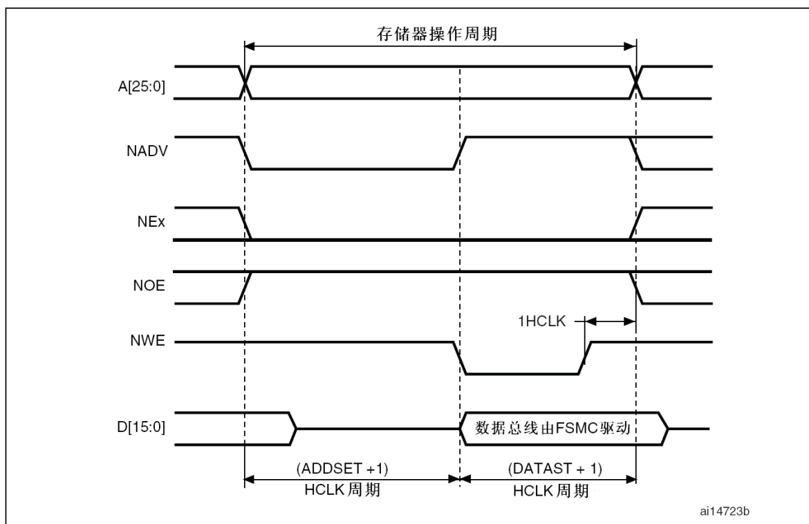
图167 模式2写操作
