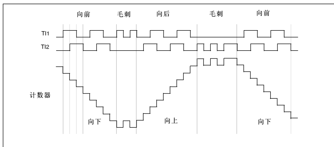
图92 IC1FP1反相的编码器接口模式实例
