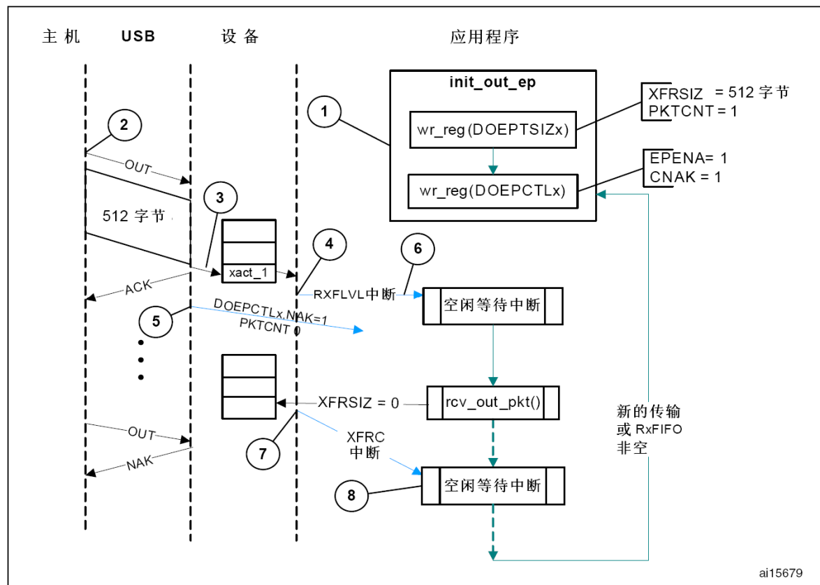
图290 从模式块(Bulk)OUT传输过程
