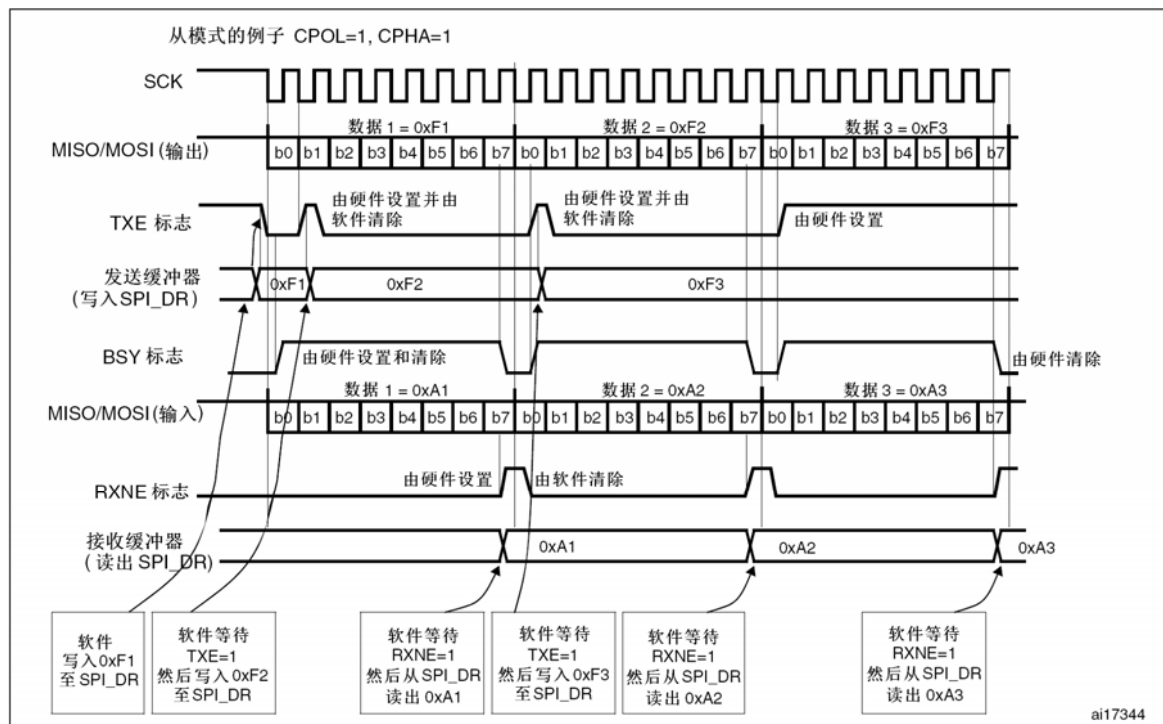
图214 从模式、全双工模式下(BIDIMODE=0并且RXONLY=0)连续传输时, TXE/RXNE/BSY的变化示意图
