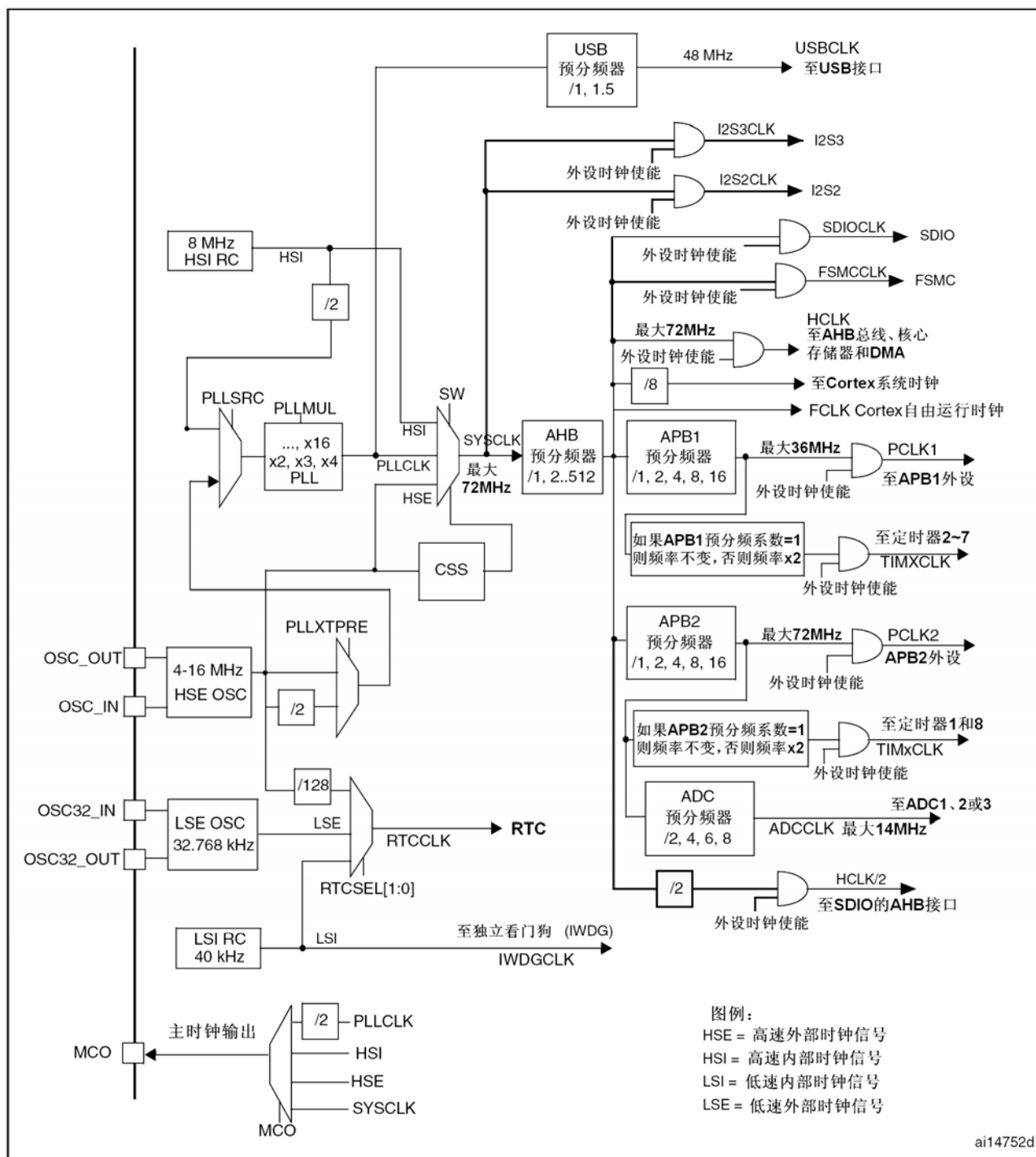
图8 时钟树
