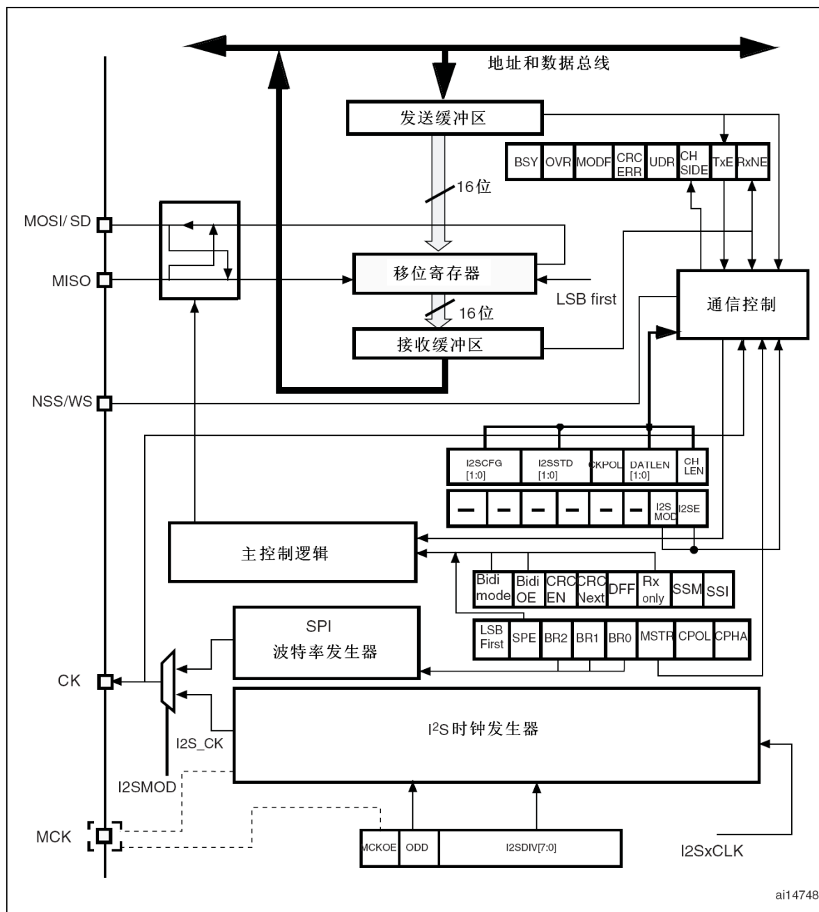
图221 I^2S 框图
