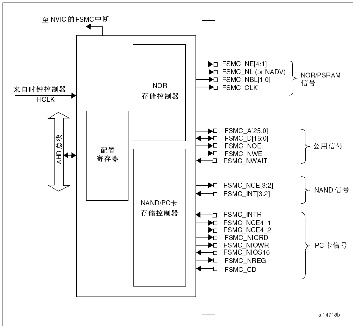
图160 FSMC框图
