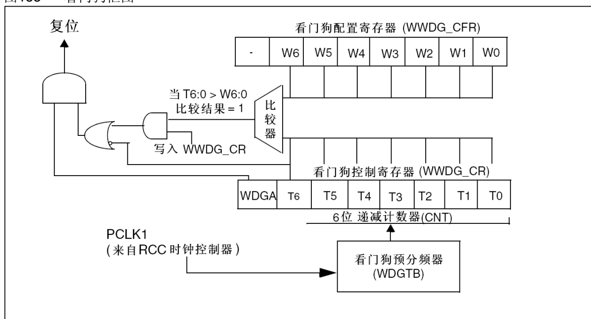
图158 看门狗框图
