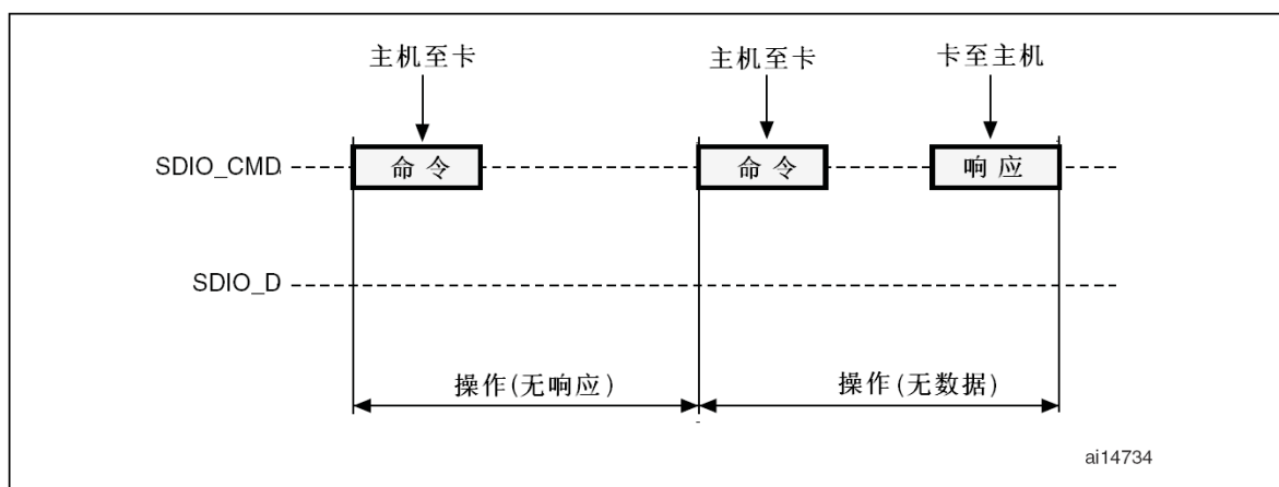
图180 SDIO(多)数据块读操作
