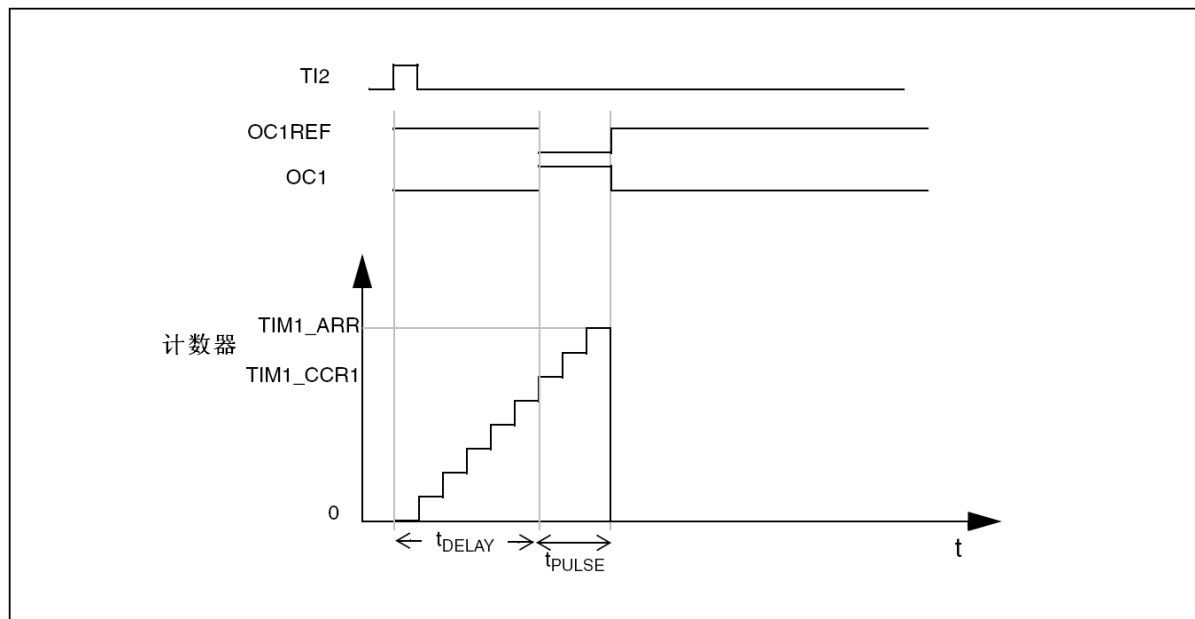
图90 单脉冲模式的例子
