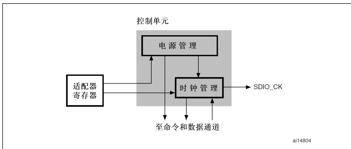
图186 控制单元
