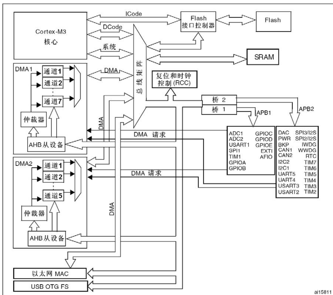
图21 DMA框图
