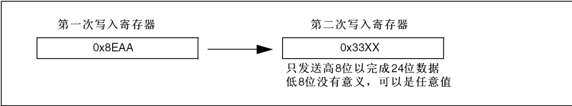
图224 发送0x8EAA33
