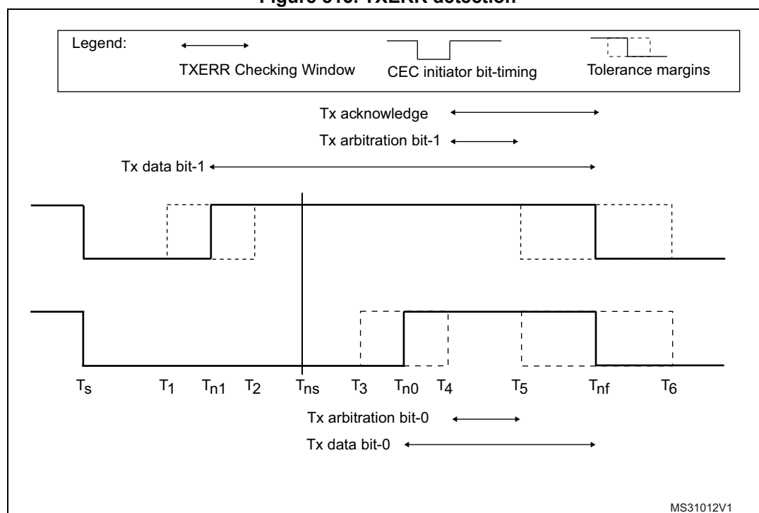
Figure 815. TXERR detection
