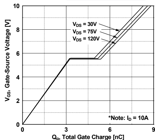
图 6. 栅极电荷
