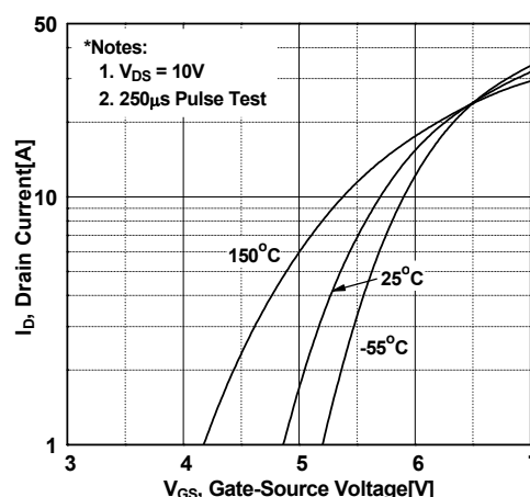
图 2. 传输特性
