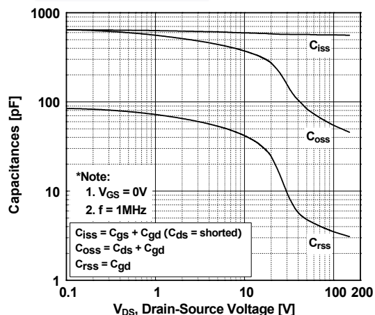
图 5. 电容特性
