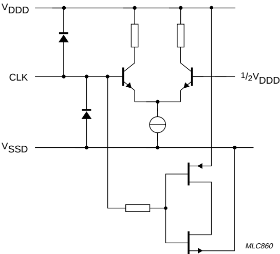
Fig.14 CLK input.
